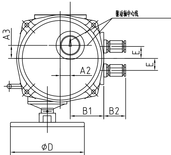
QT1Ex~QT4Ex系列外形尺寸
