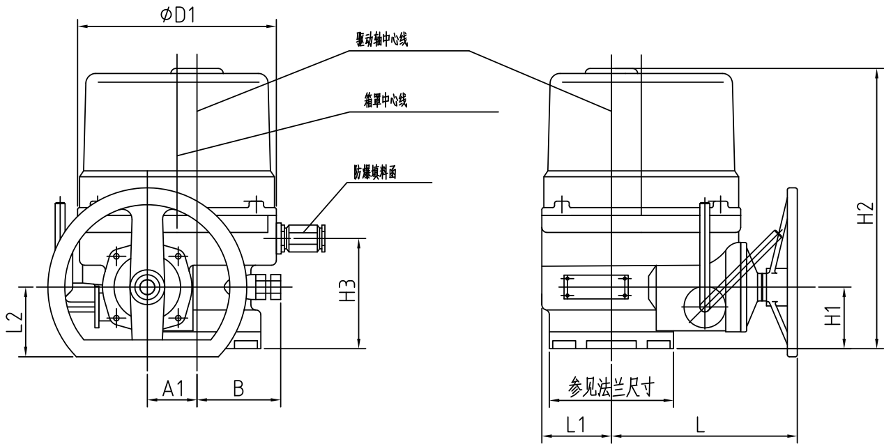
防爆填料函
